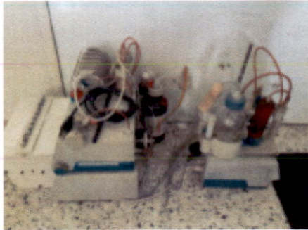
ชื่อ : Karl Fischer Titration Set
